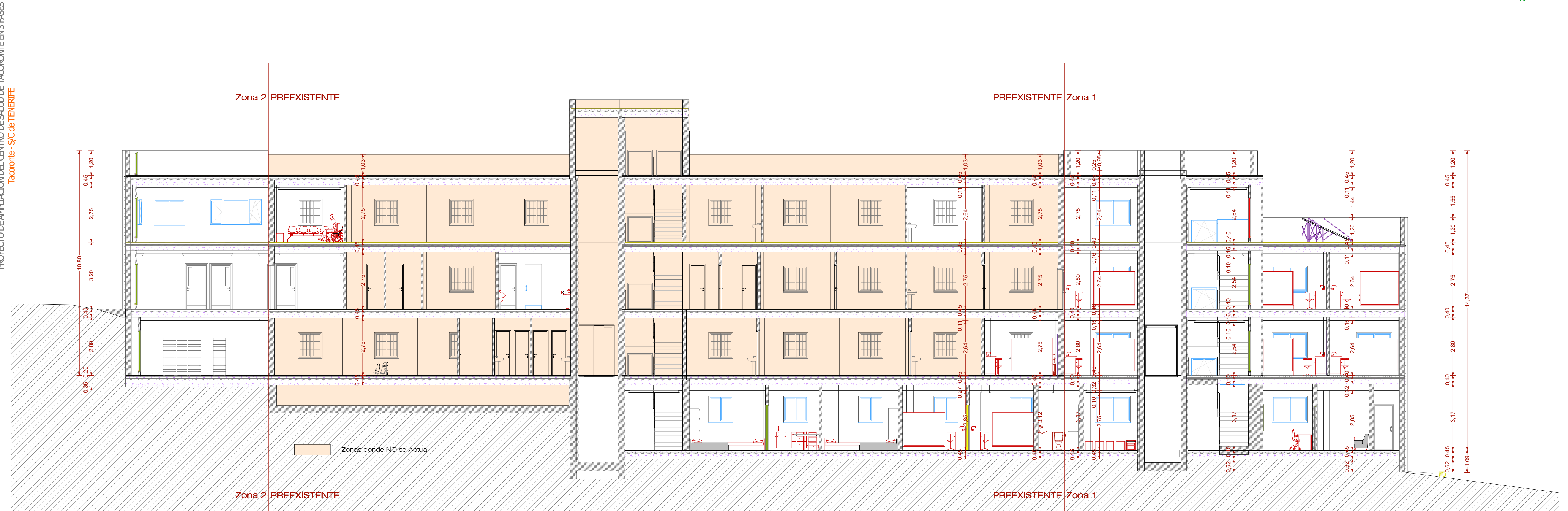
Sección Longitudinal 4
