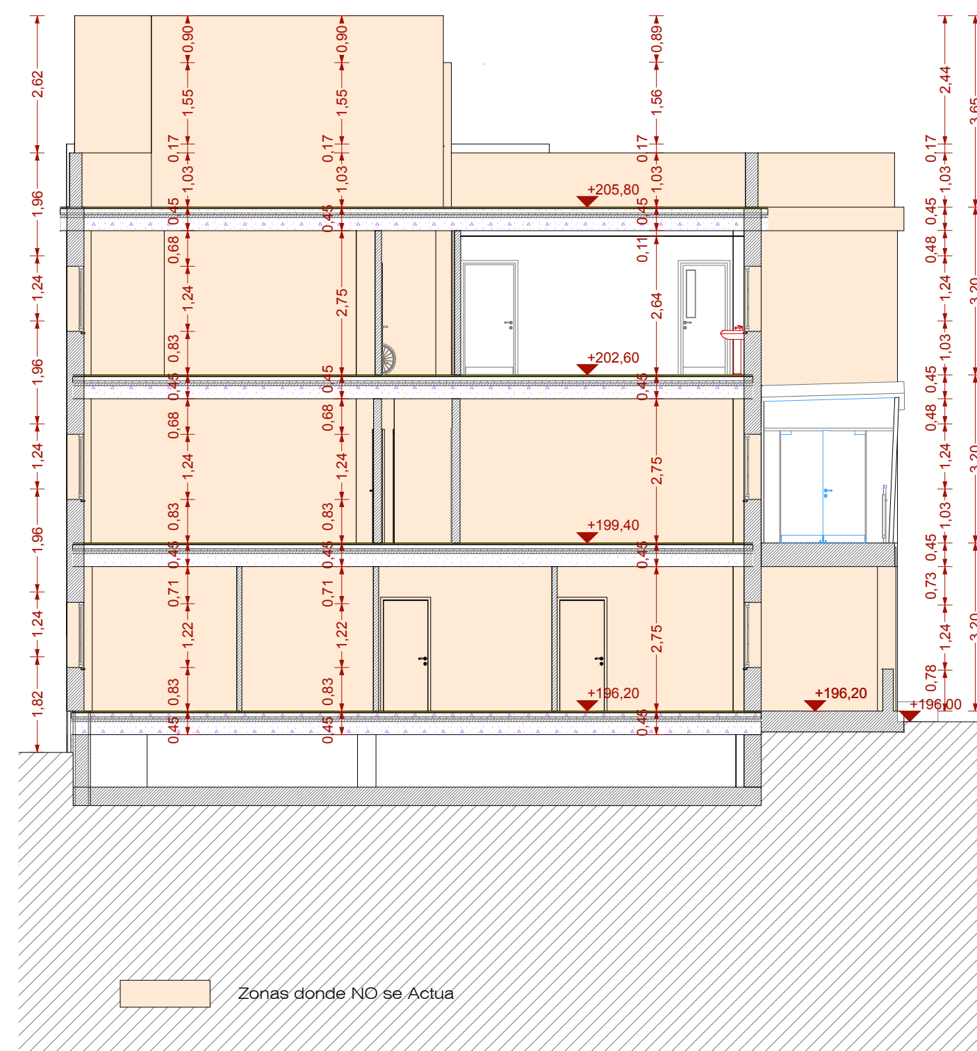
Sección Transversal 2
