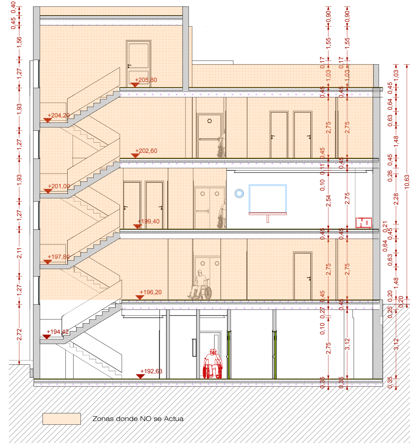
Sección Transversal 3
