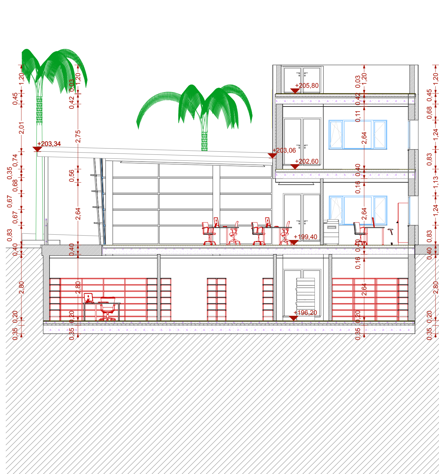
Sección Transversal 1
