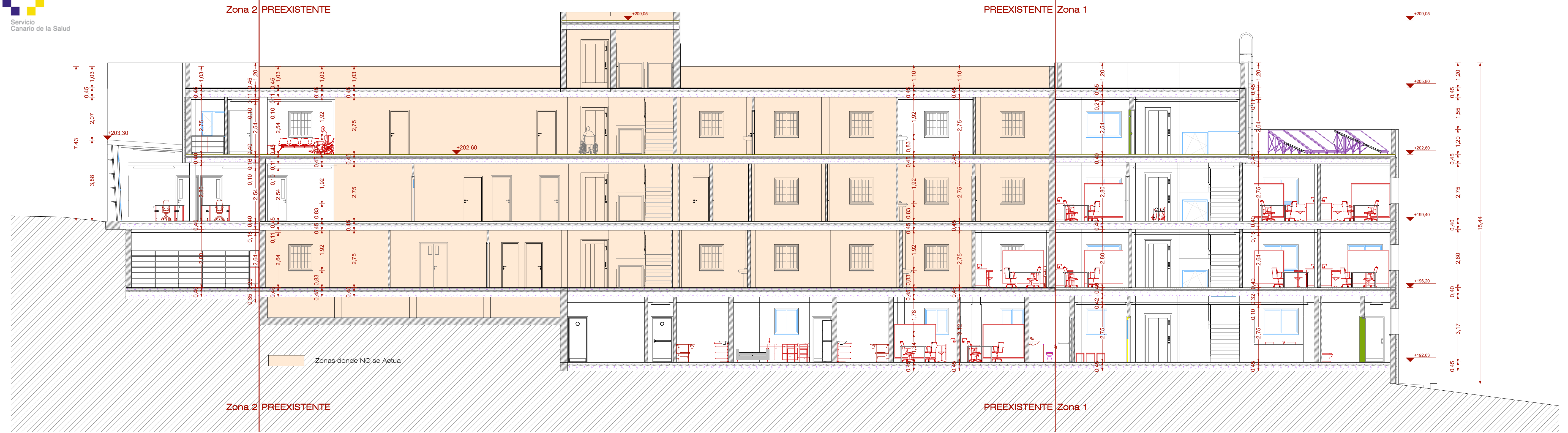
Sección Longitudinal 3
