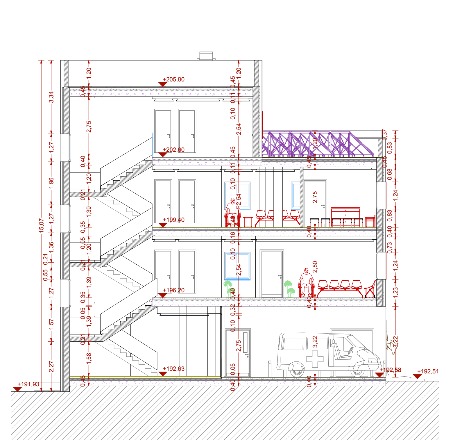
Sección Transversal 4
